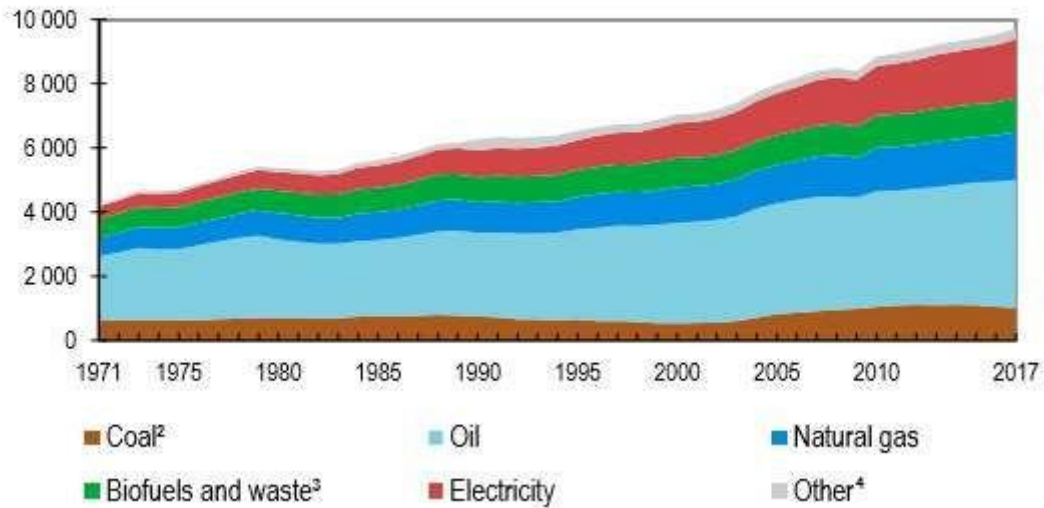
Figure 2 – Evolution de la consommation mondiale d'énergie
