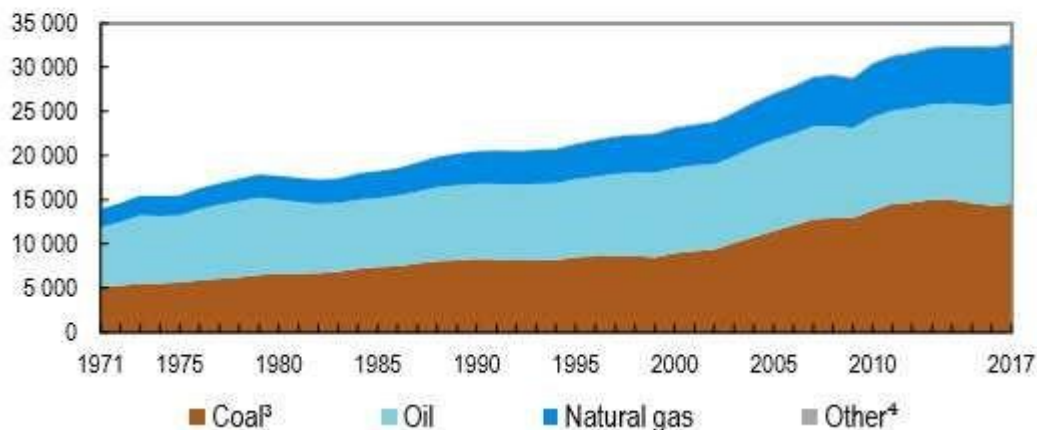
Figure 5 – Evolution des émissions de CO 2 par type de combustible (millions de t de CO 2 )
