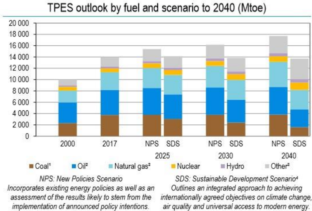
Figure 3 – Evolution de la production d'énergie primaire en Mtep par type de source d'énergie
