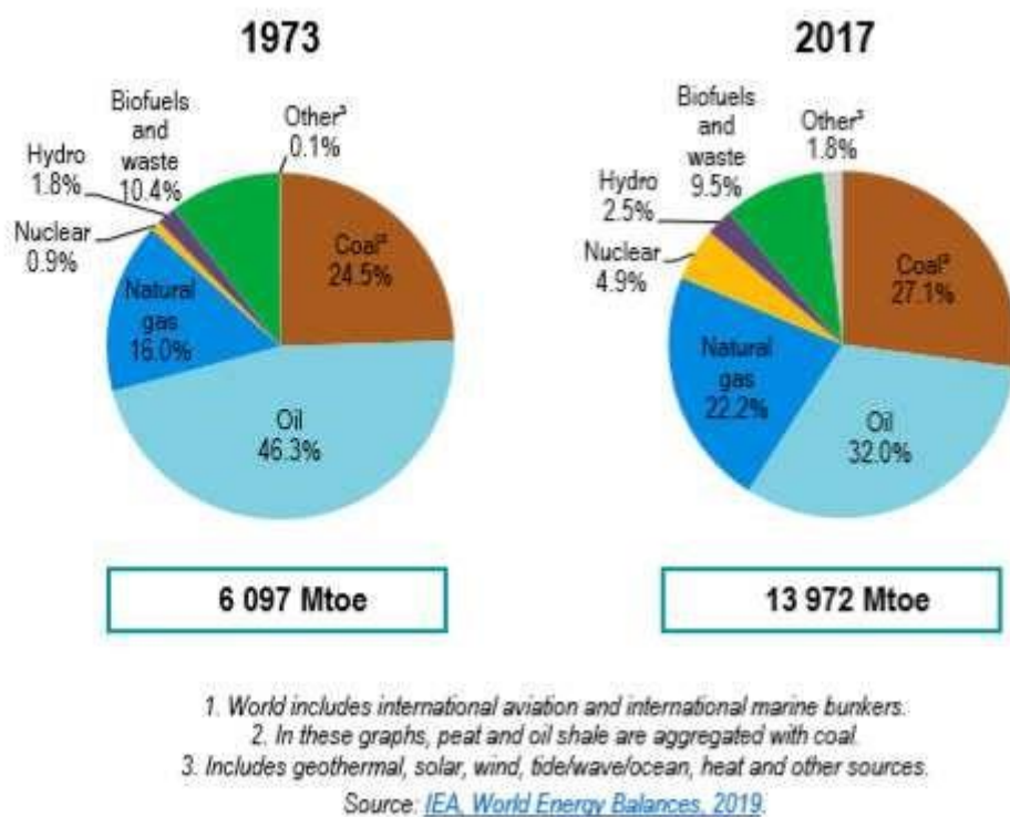
Figure 1 – Evolution de la production d'énergie primaire (en millions de toe: ton of oil equivalent, 1 toe = 1 tep) par source
