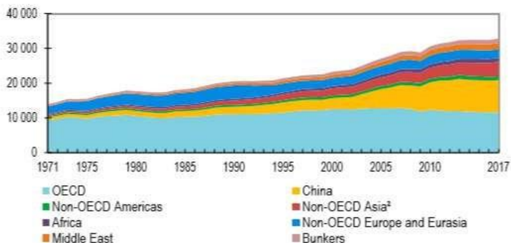
Figure 6 – Evolution des émissions de CO 2 par zone économique (millions de t de CO 2 ) Source:
