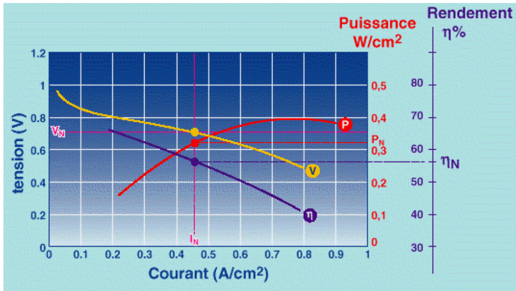
Fig. 3 – Caractéristiques électriques de la pile PEM
