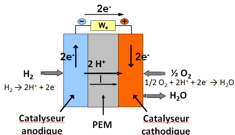
Fig. 2 - Schéma de principe d'une pile à combustible de type PEM
