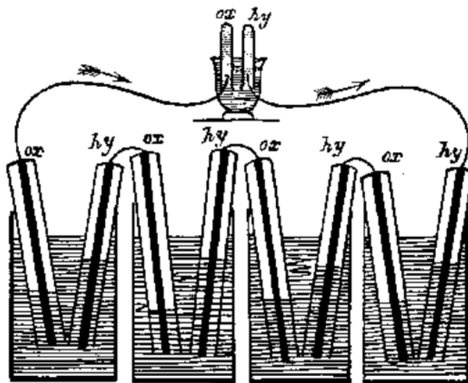
Figure 1 - Schéma de la première pile à combustible de William Grove (1839)
